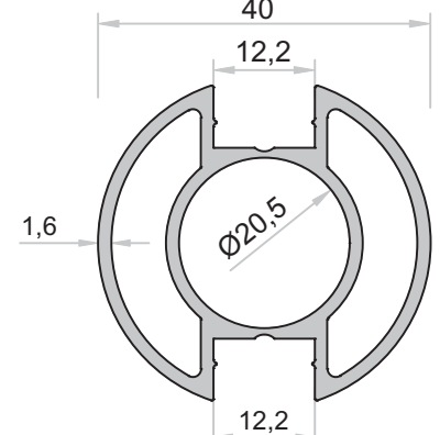
4279 - 0,854 kg/m
