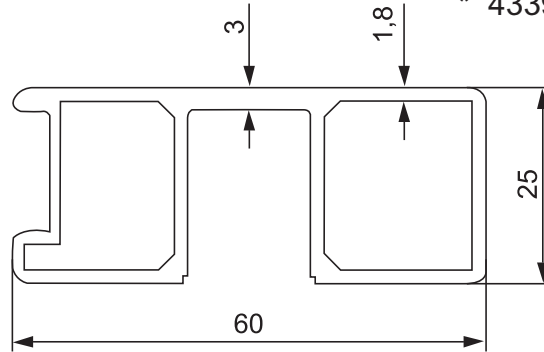
9033 - 991 gr/m
