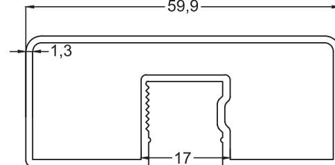
2558 0.693 Kg/m
