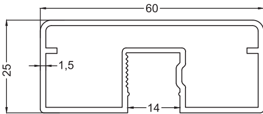
156 0.802 Kg/m
