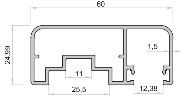
* 4339 - 0,781 kg/m
