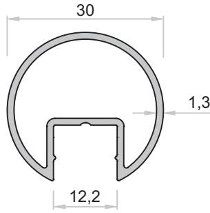
3580 - 0,387 kg/m
