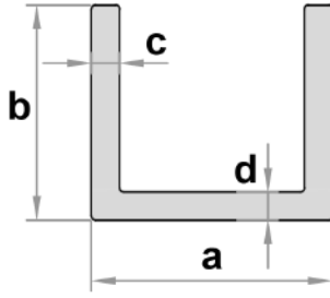
U-PROFİLLERİ U-FILES
