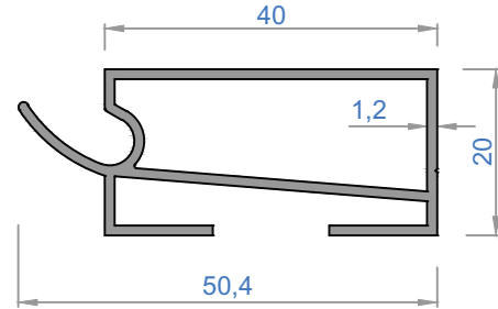
4392 - 0,504 kg/m
