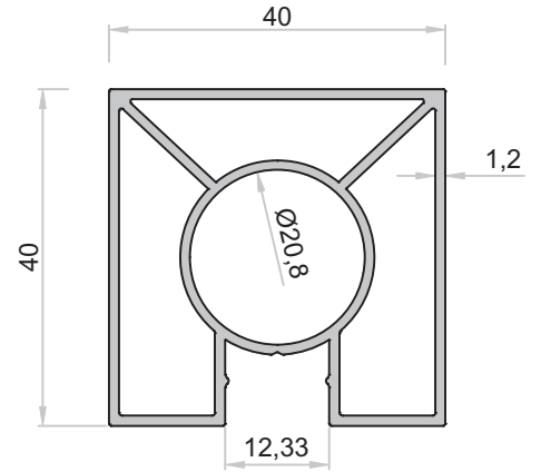
3818 - 0,874 kg/m
