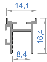
4232 - 0,160 kg/m
