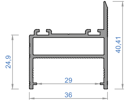
5791 - 0,595 kg/m
