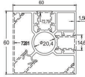
* 7272 60x60 Çit Dikme Profili 1,376 kg/mt
