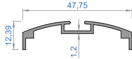
1093 - 0,295 kg/m
