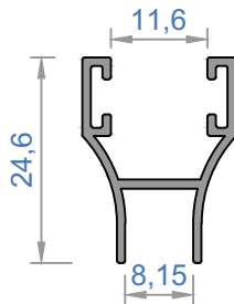
4825 - 0,210 kg/m
