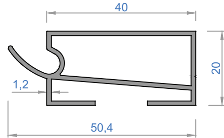
4392 - 0,504 kg/m
