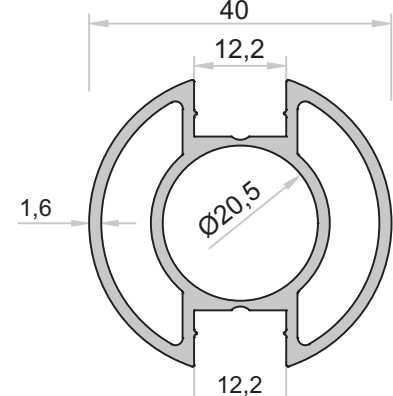
4279 - 0,854 kg/m
