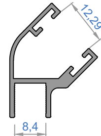
4393 - 0,277 kg/m
