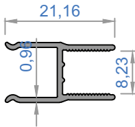
3974 - 0,150 kg/m
