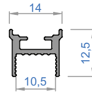
* 4438 - 0,130 kg/m
