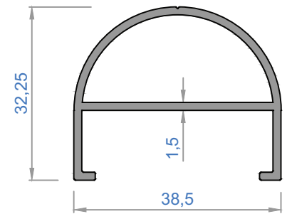
* 4382 - 0,506 kg/m
