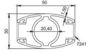
* 7803 30x50 Elips Çift Kanal Dikme Profili 1,149 kg/mt
