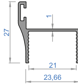
5425 - 0,246 kg/m
