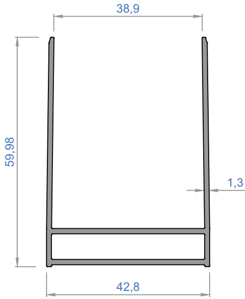
5412 - 0,727 kg/m
