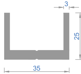
2577 - 0,800 kg/m
