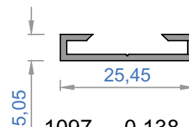
1097 - 0,138 kg/m
