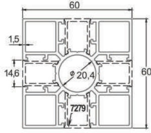
* 7271 60x60 Çit Dikme Profili 1,937 kg/mt
