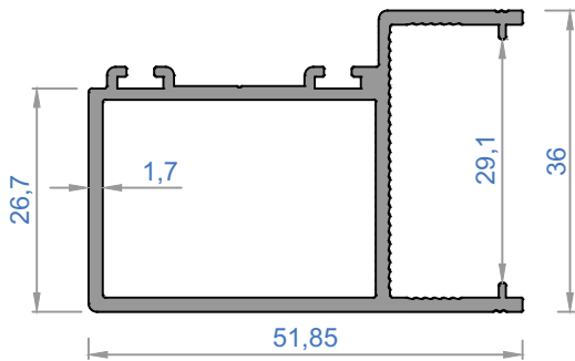
5786 - 0,757 kg/m
