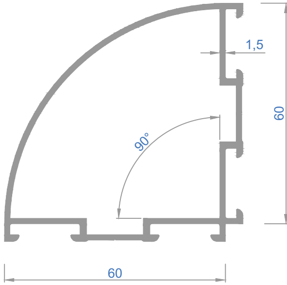
1248 - 1,106 kg/m
