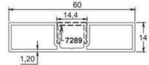
* 7277 60x14 Çit Profili 0,523 kg/mt
