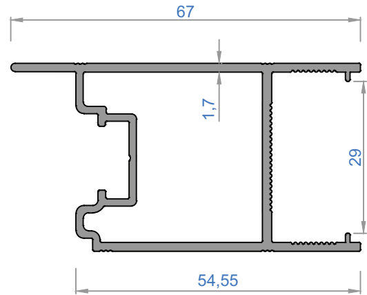
5793 - 0,905 kg/m
