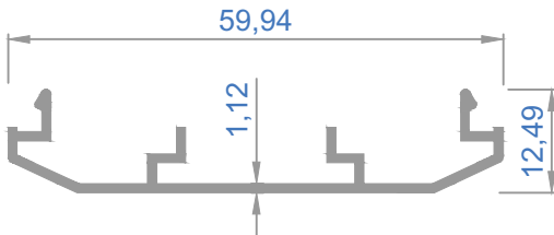
2580 - 0,324 kg/m
