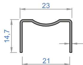
5423 - 0,136 kg/m
