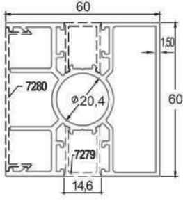
* 7270 60x60 Çit Dikme Profili 1,639 kg/mt
