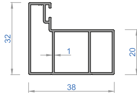
4389 - 0,480 kg/m
