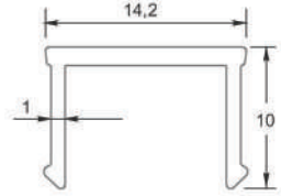
* 7289 Kapak (7277 Profil Kapağı) 0,098 kg/mt
