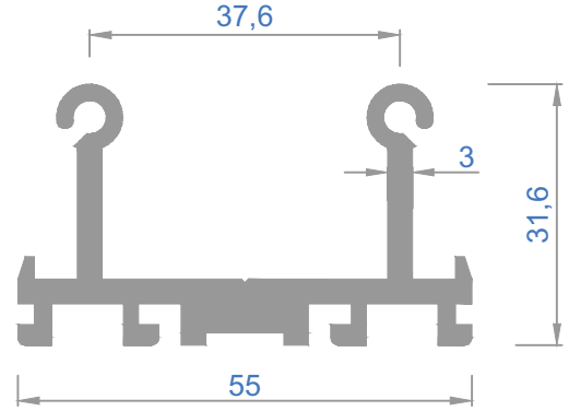
1247 - 1,238 kg/m
