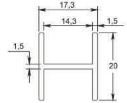
* 7278 20x17,3 Çit Profili 0,220 kg/mt
