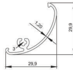
* 7806 30x30 Elips Profil Kapağı 0,243 kg/mt
