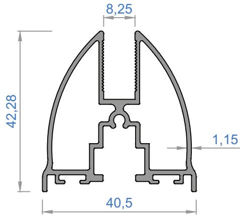
5209 - 0,736 kg/m
