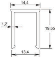
* 7279 Kapak 0,175 kg/mt
