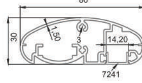
* 7802 30x80 Elips Profil 1,221 kg/mt
