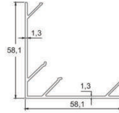
* 7281 Kapak 0,580 kg/mt
