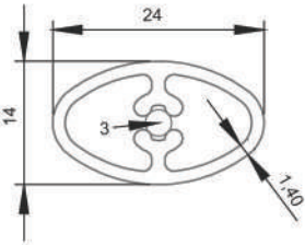
* 7808 14x24 Elips Profil 0,289 kg/mt
