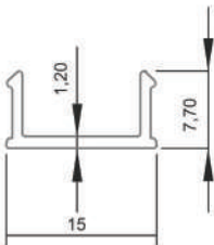
* 7241 30x50 Dikme Kapağı 0,084 kg/mt
