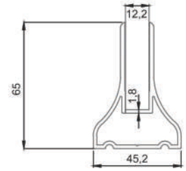
* 4892 Alt Etek Profili Çiftli 1,196 kg/mt
