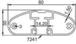
* 7800 30x80 Elips Profil 1,221 kg/mt
