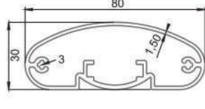
* 7801 30x80 Elips Profil 1,099 kg/mt
