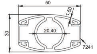
* 7803 30x50 Elips Çift Kanal Dikme Profili 1,149 kg/mt
