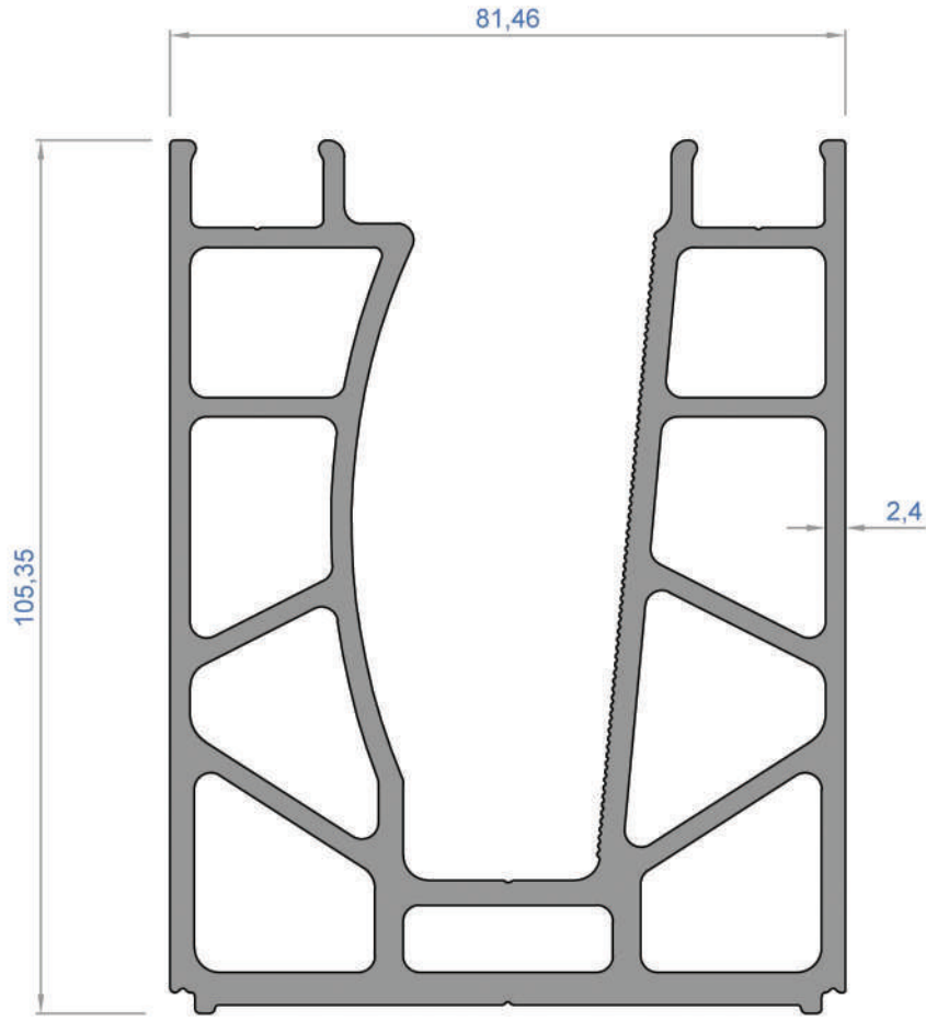
4800 - 5,322 kg/m
