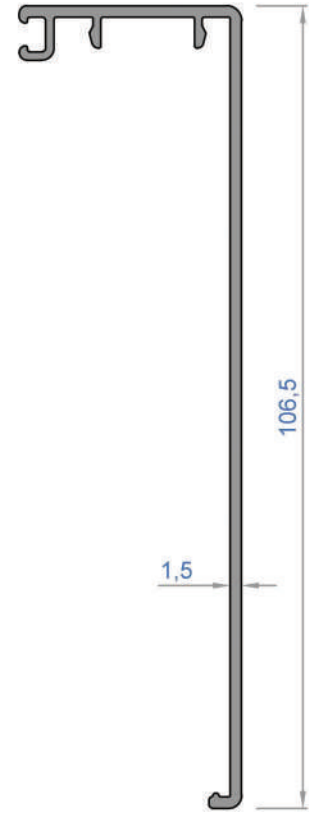
4801 - 0,607 kg/m
